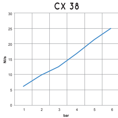
不同供应压力 (bar) 下的空气消耗量 (NI/s)
